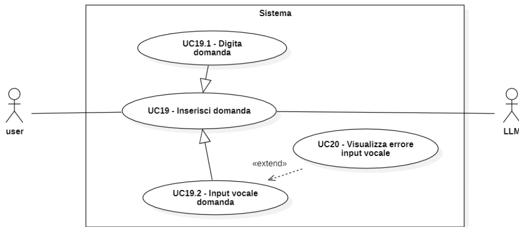
Figura 23: Diagramma UML dei casi d'uso UC-19, UC-19.1, UC-19.2 e 20
