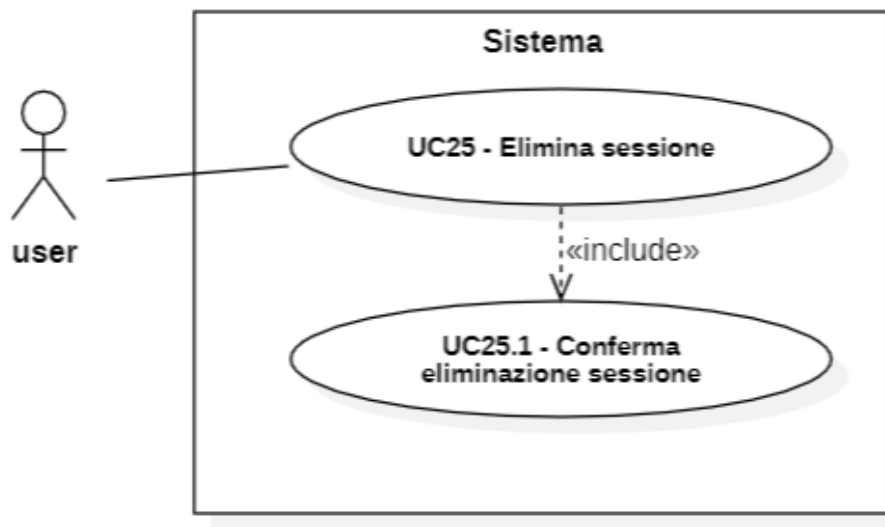
Figura 28: Diagramma UML dei casi d'uso UC-25 e UC-25.1
