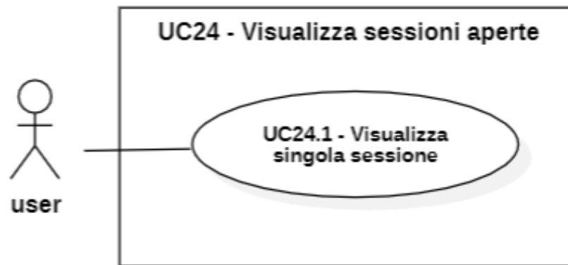
Figura 27: Diagramma UML del caso d'uso UC-24.1
