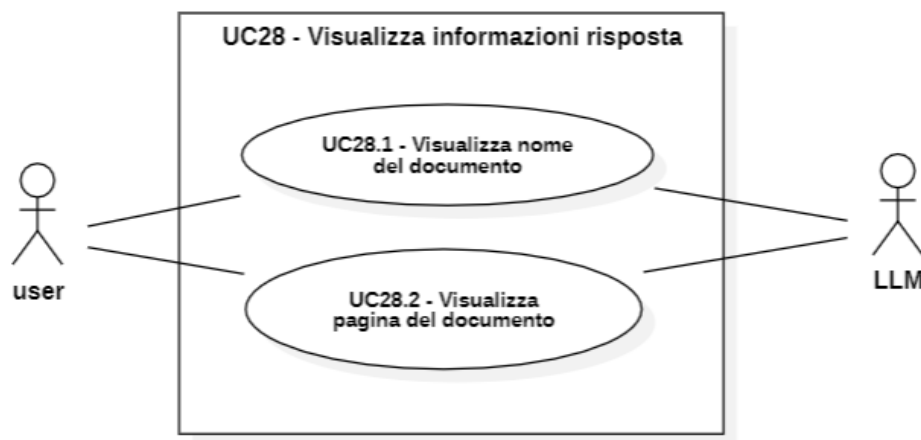
Figura 32: Diagramma UML dei casi d'uso UC-28.1 e UC-28.2
