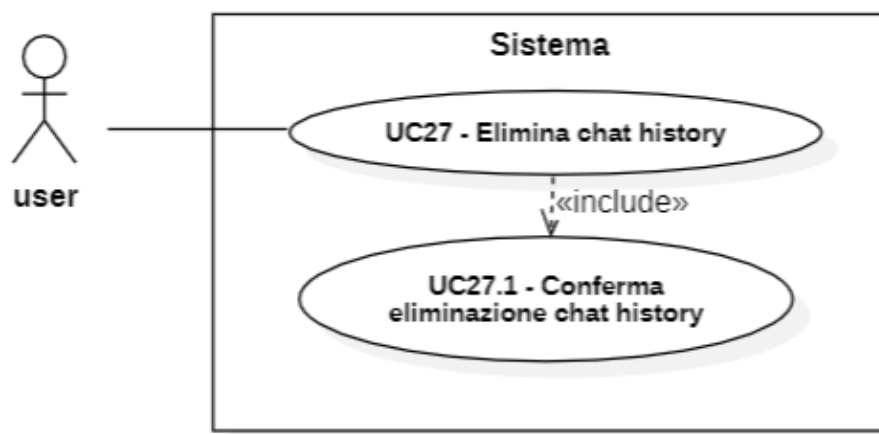
Figura 30: Diagramma UML dei casi d'uso UC-27 e 27.1
