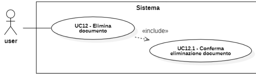
Figura 17: Diagramma UML dei casi d'uso UC-12 e UC-12.1
