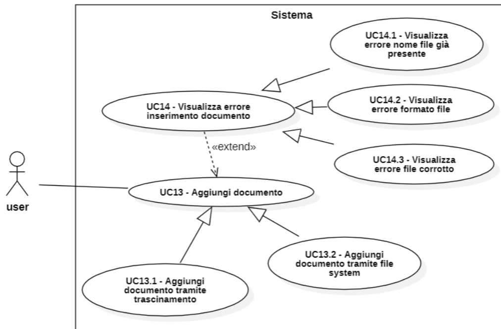
Figura 18: Diagramma UML dei casi d'uso UC-13, UC-13.1, UC-13.2, UC-14, UC-14.1, UC-14.2 e UC-14.3
