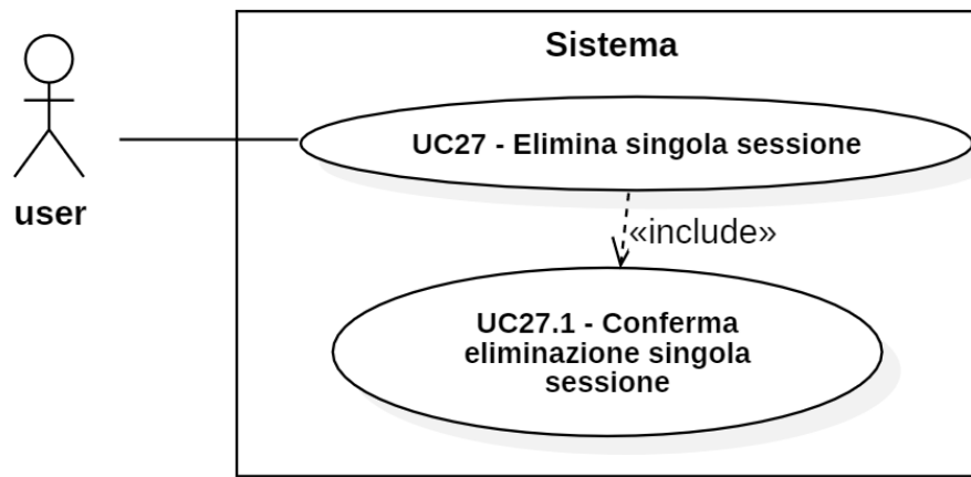
Figura 32: Diagramma UML dei casi d'uso UC-27 e UC-27.1
